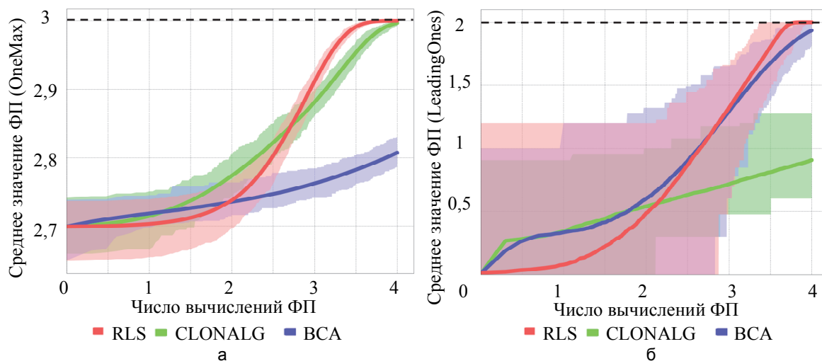
Рис. 1. Зависимость среднего значения функции приспособленности от числа ее вычислений алгоритмами RLS, BCA и CLONALG на задачах OneMax (а) и LeadingOnes (б). Значения по обеим осям логарифмированы по основанию 10
